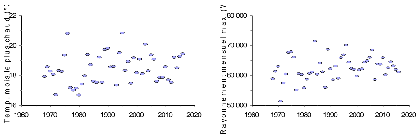
Figure 8 : Evolution des températures moyennes et de l'ensoleillement cumulé pour les mois les plus chauds (90 ème centile) depuis 1968 à Nort sur Erdre
